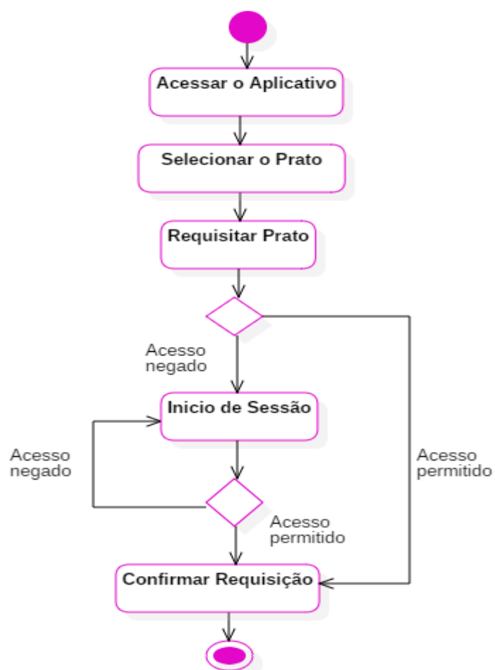
Figura 2: Diagrama de actividades da requisição;
