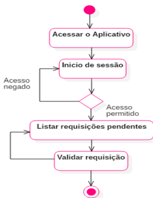
Figura 4: Diagrama de Actividade de Validação de Requisição;
