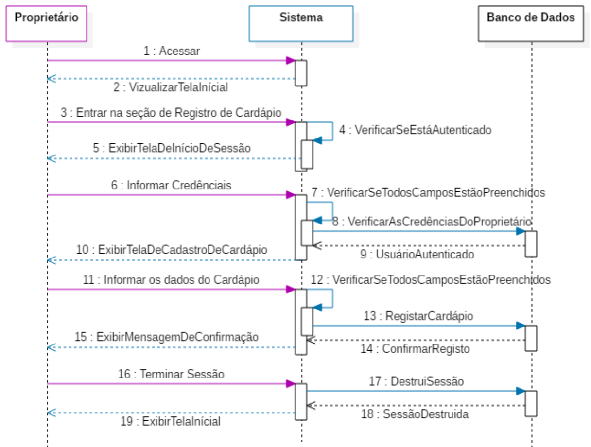
Figura 6: Diagrama de Sequência de registo de Cardápios;
