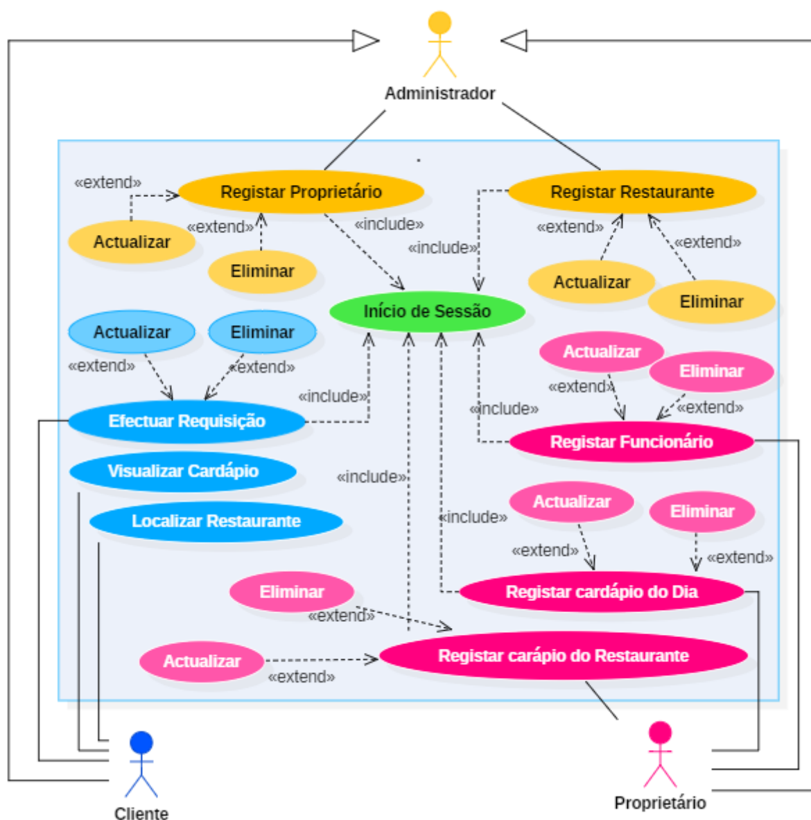
Figura 1: Diagrama de caso de uso do sistema;
