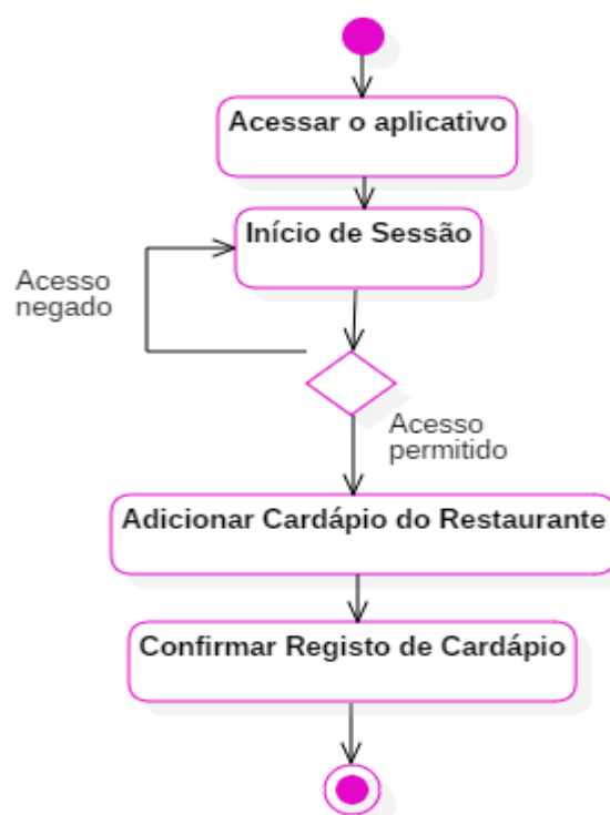
Figura 3: Diagrama de actividades do registo de cardápio;
