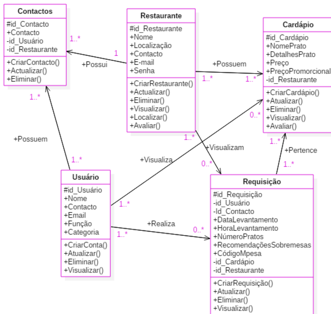
Figura 8: Diagrama de Classe do aplicativo;
