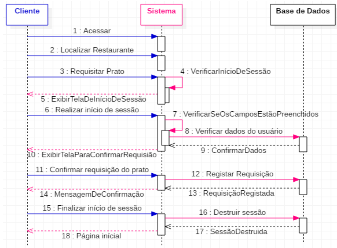
Figura 5: Diagrama de Sequência de Requisição de um Prato;
