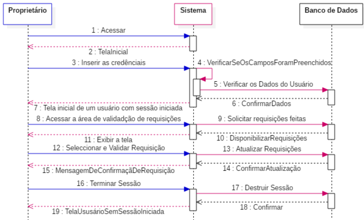
Figura 7: Diagrama de Sequência de Validação de Requisição;
